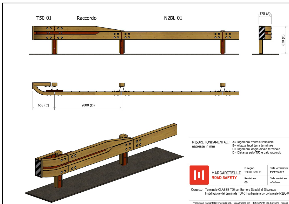
Figura 6 Connessione con N2BL-01
