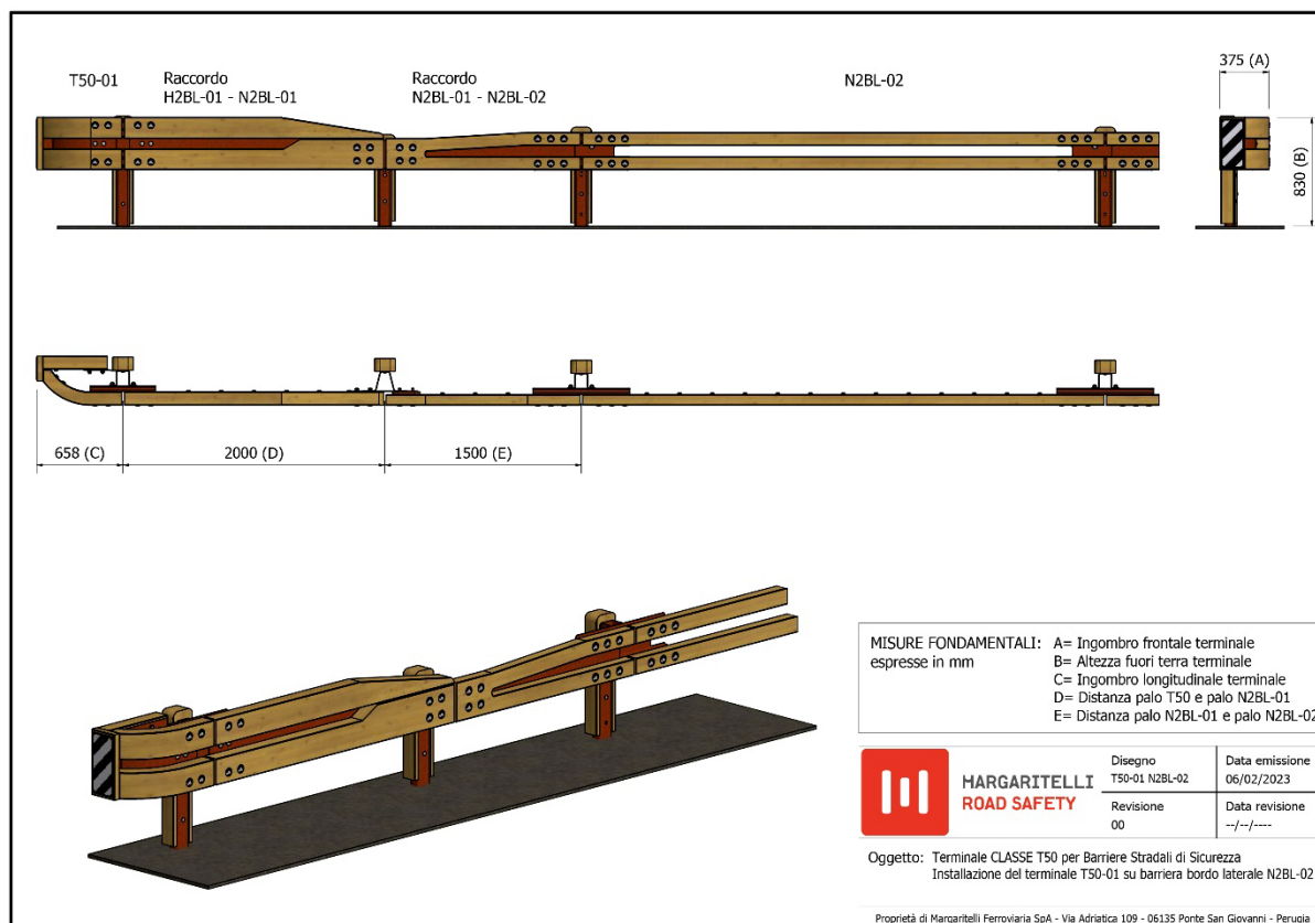
Figura 7 Connessione con N2BL-02
