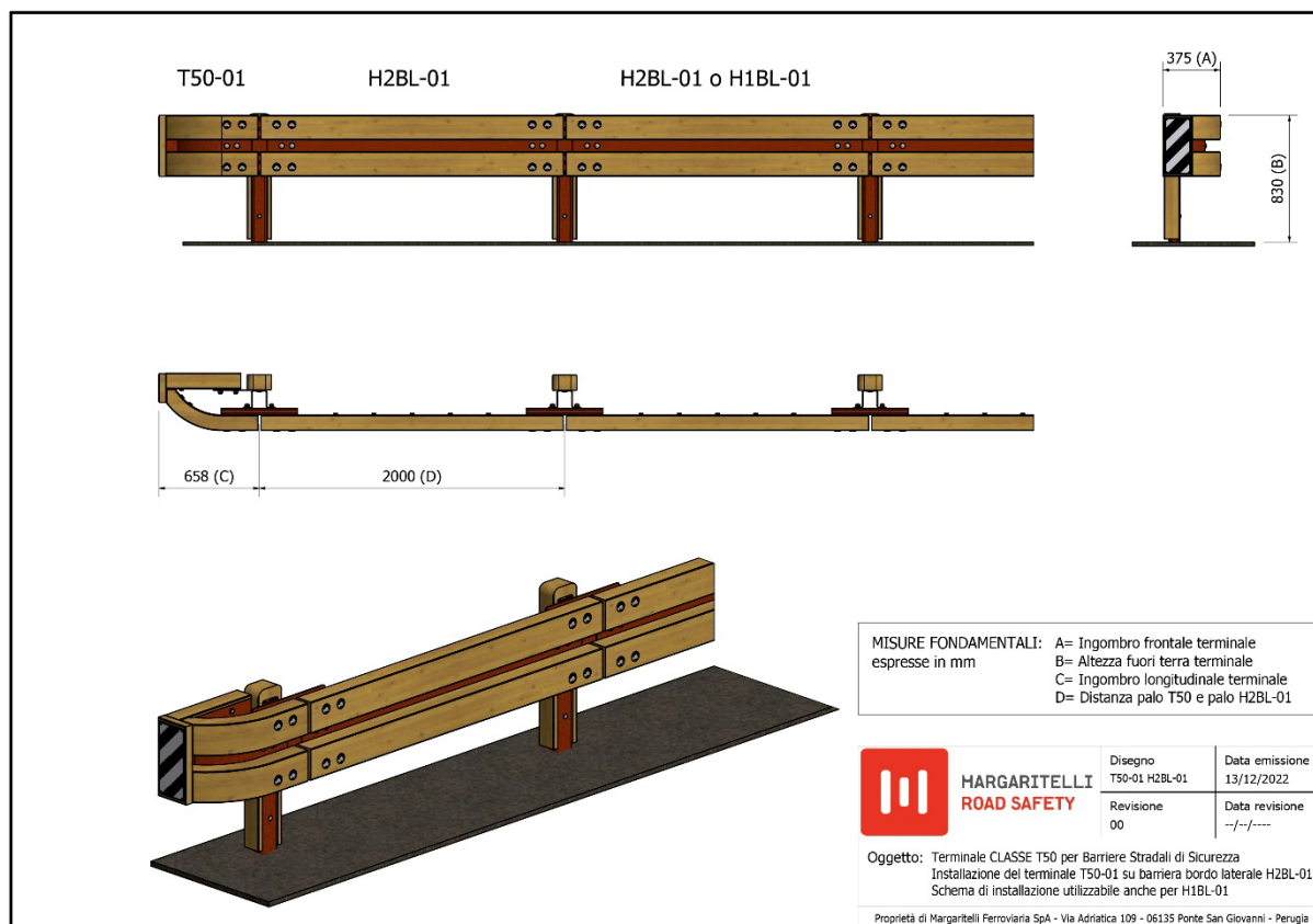
Figura 5 Connessione con H2BL-01 o H1BL-01
