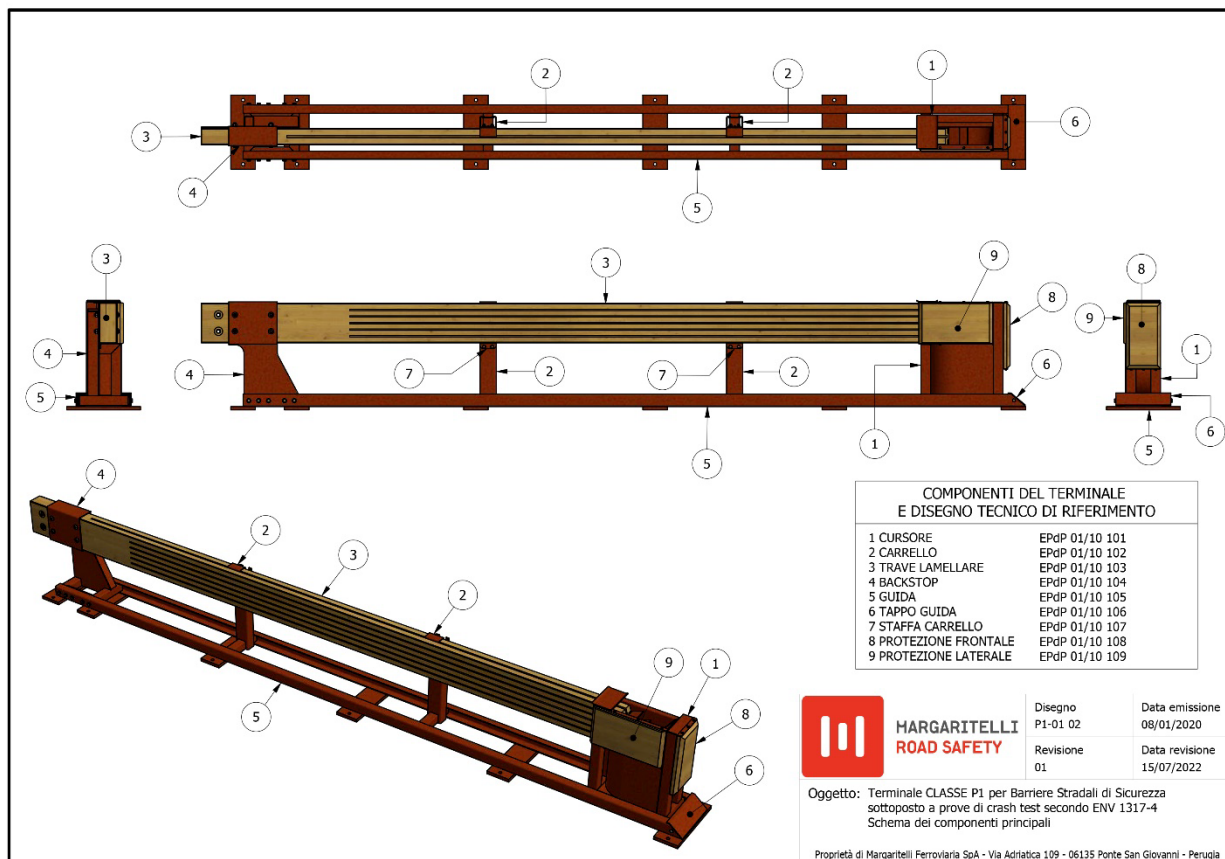
Figura 7 Componenti principali
