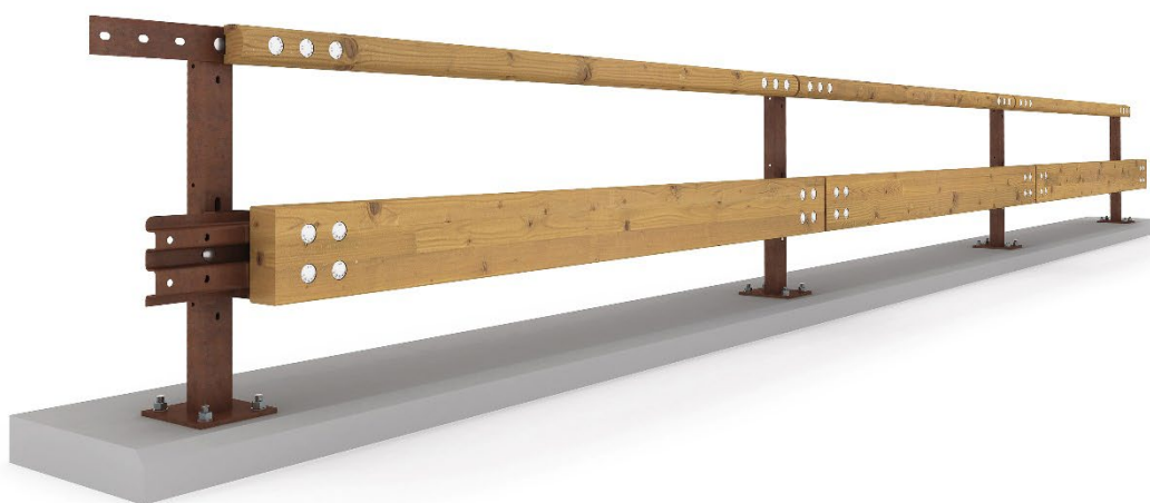
Figura 2 Trattamento superficiale trasparente, colore naturale - Nessun rivestimento del palo
