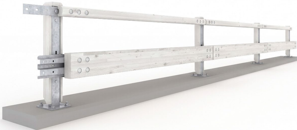
Figura 4 Su richiesta trattamento superficiale bianco con acciaio zincato
