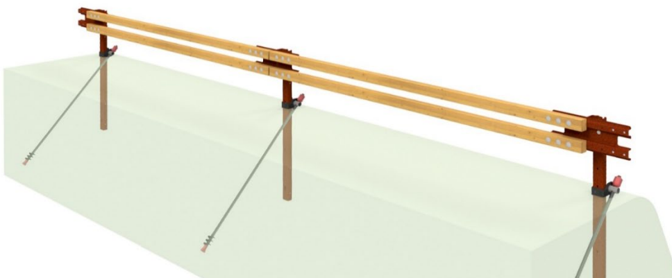
Figura 12 schema della barriera N2BL-02 integrata con sistema ASDR-MRS
