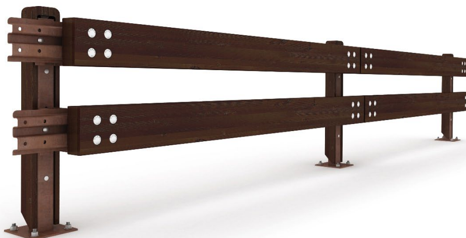
Figura 2 Su richiesta trattamento superficiale colore noce
