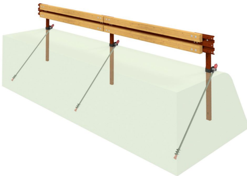
Figura 13 schema della barriera H1BL-01 integrata con sistema ASDR-MRS
