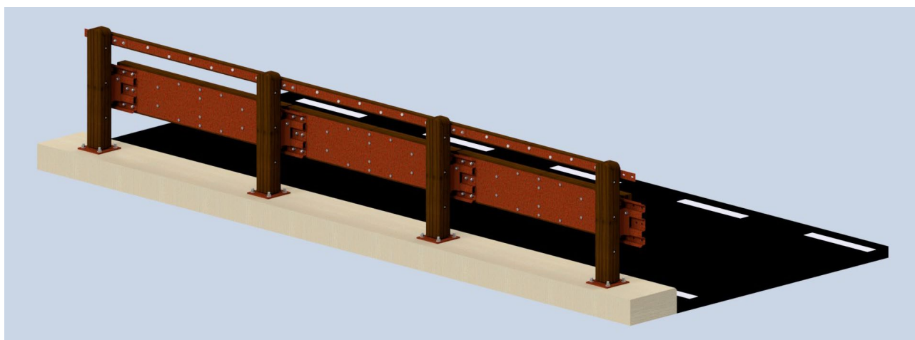
Figura 8 Vista posteriore della barriera con trattamento superficiale colore noce scuro
