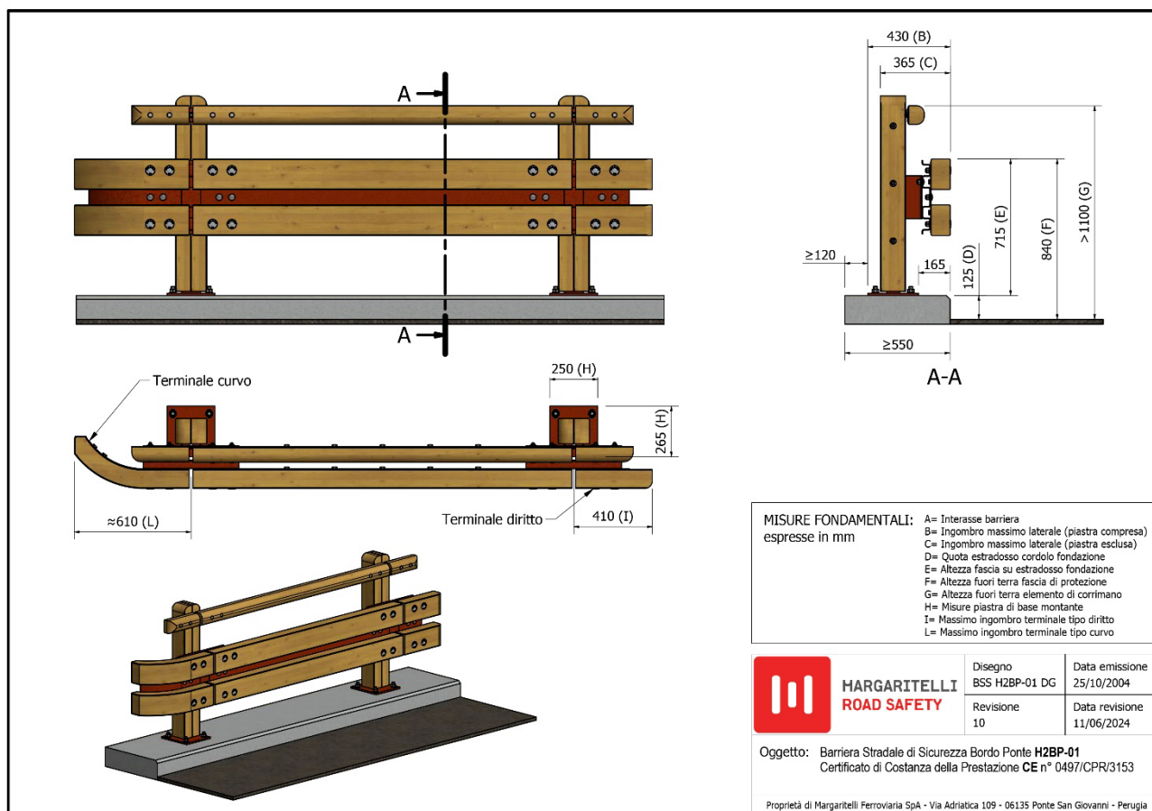
Figura 4 schema della barriera in versione standard
