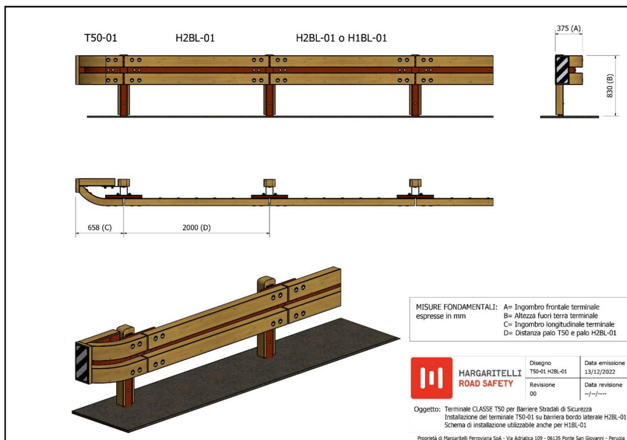
Figura 6 schema di collegamento tra barriera bordo laterale e terminale T50-01
