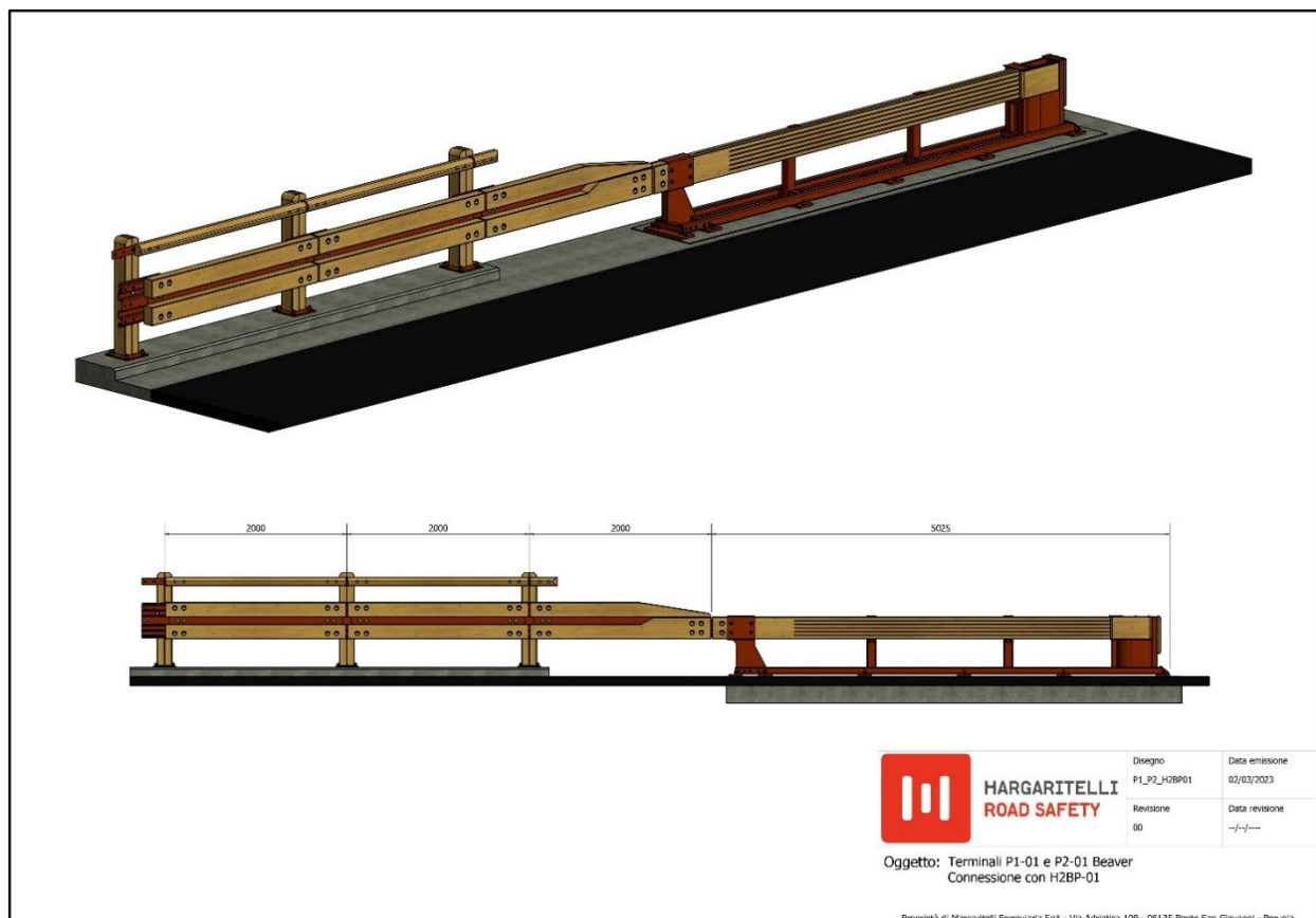
Figura 5 schema della barriera con collegamento diretto con terminale P1-01 o P2-01 Beaver
