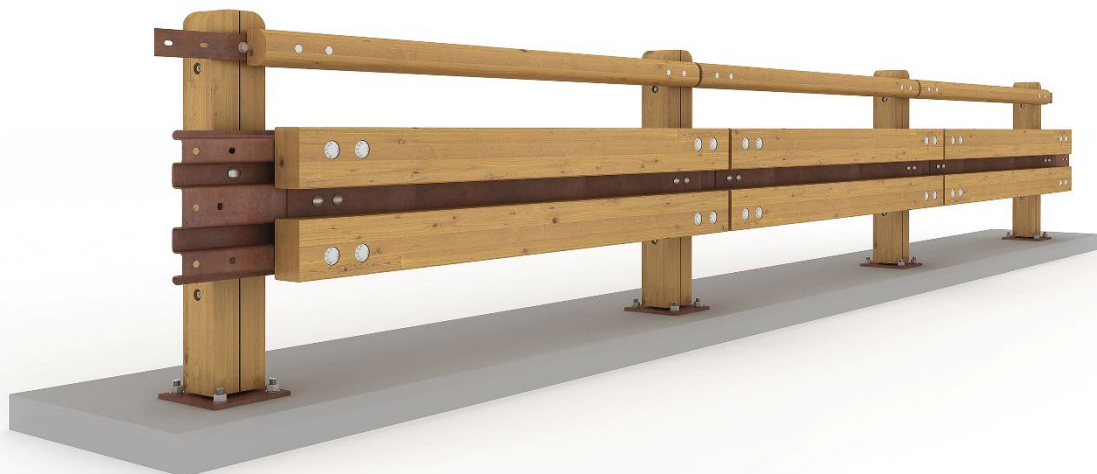
Figura 1 Trattamento superficiale trasparente, colore naturale - Doppio guscio di rivestimento del palo
