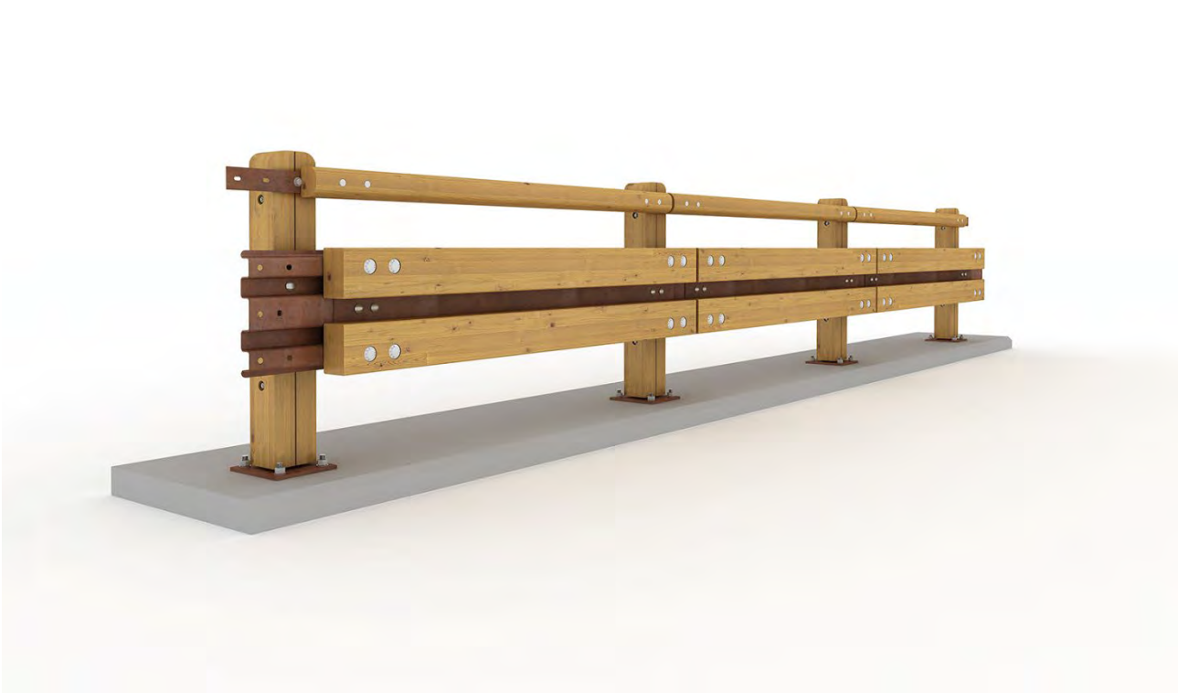
Figura 1 – Barriera con singolo guscio di rivestimento del montante
