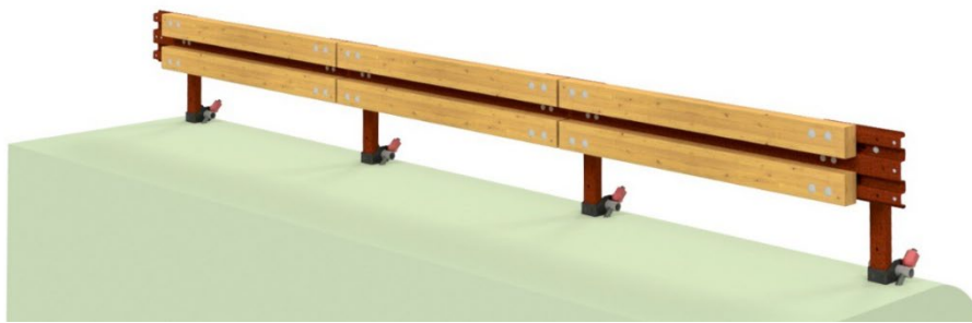
Figura 5.5 - Barriera H2BL-01 dotata di sistema ASDR-MRS
