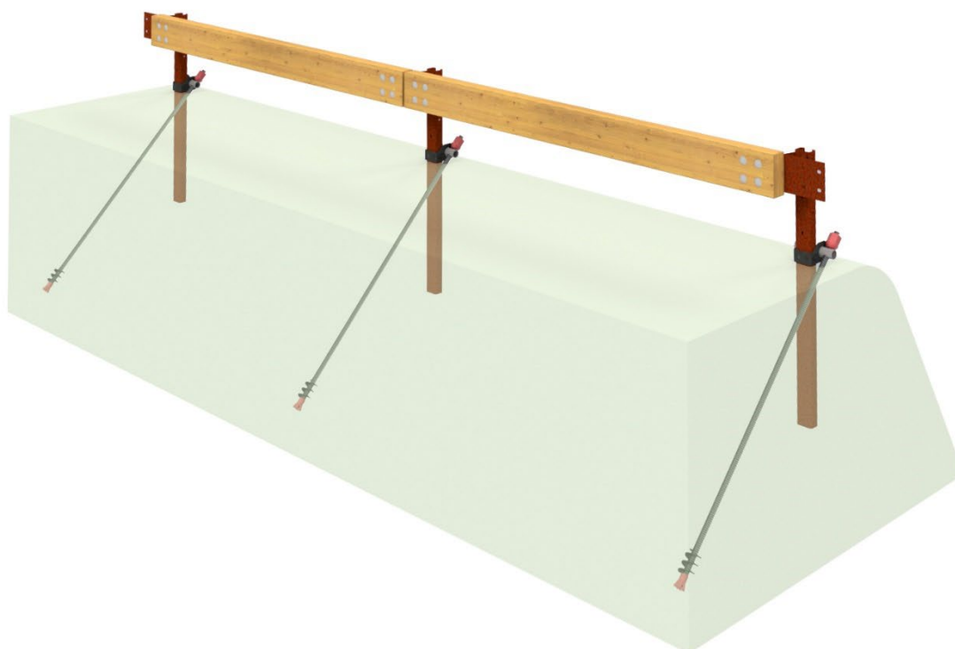
Figura 5.3 - Barriera N2BL-01 dotata di sistema ASDR-MRS con rilevato trasparente
