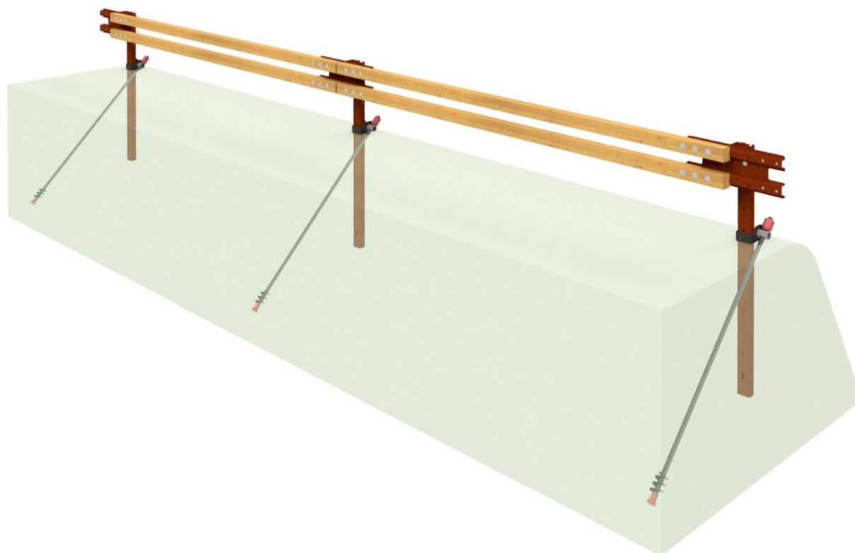
Figura 5.4 - Barriera N2BL-02 dotata di sistema ASDR-MRS con rilevato trasparente
