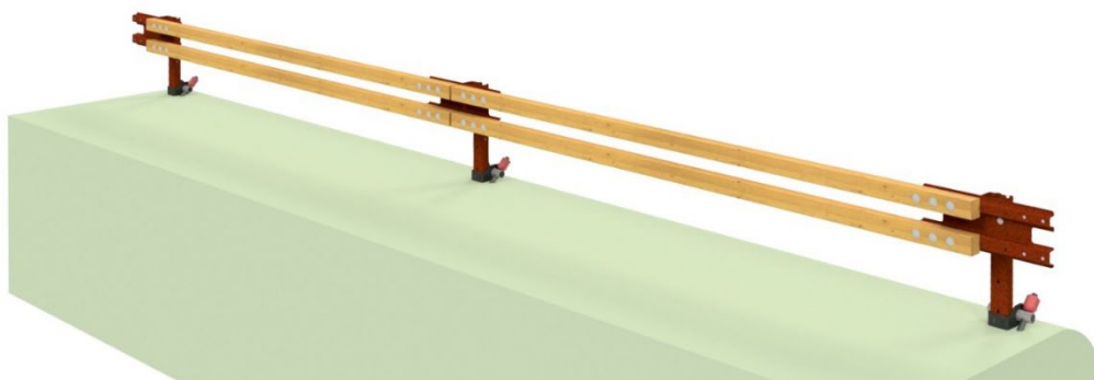
Figura 5.8 - Barriera N2BL-02 dotata di sistema ASDR-MRS
