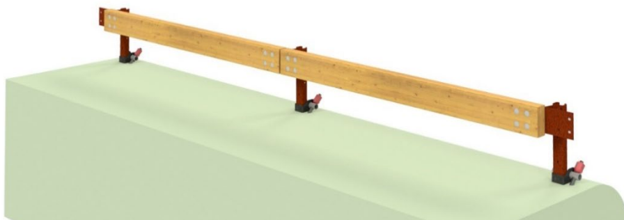
Figura 5.7 - Barriera N2BL-01 dotata di sistema ASDR-MRS
