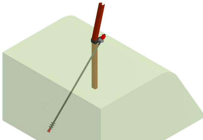
Figura 1.3. meccanismo di collasso con sistema ASDR-MRS installato
