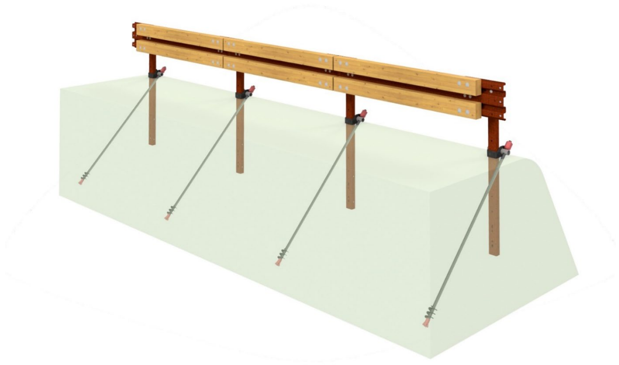
Figura 5.1 - Barriera H2BL-01 dotata di sistema ASDR-MRS con rilevato trasparente
