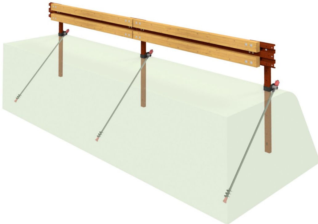
Figura 5.2 - Barriera H1BL-01 dotata di sistema ASDR-MRS con rilevato trasparente
