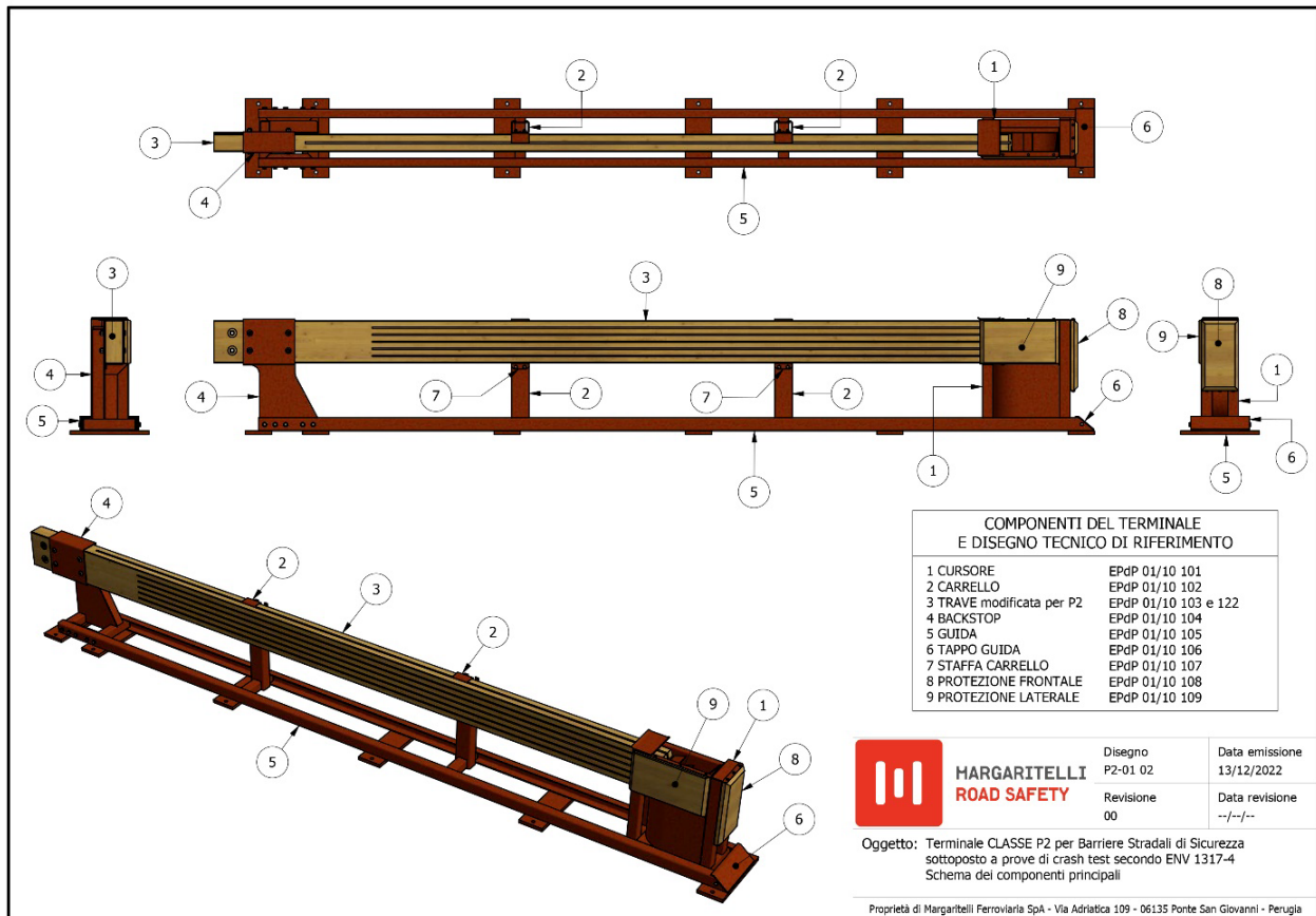
Figura 7 Componenti principali
