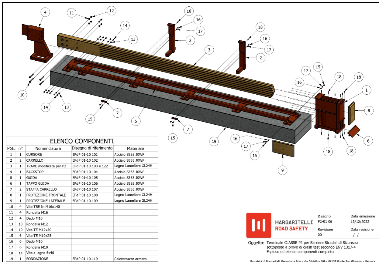
Figura 8 Esploso
