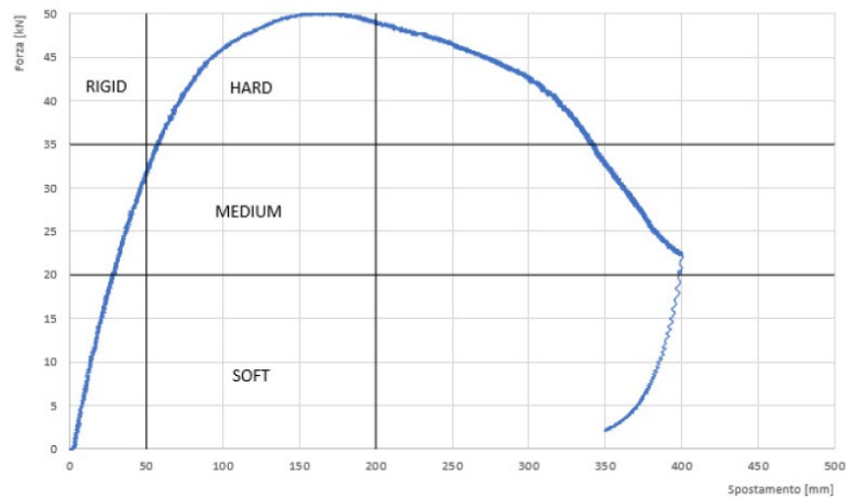
Figura 6 – risultato della prova di push quasi statico con HEB 120 con infissione di 1 metro
