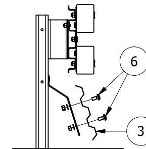
Fase "B" - Installazione piastra di continuità
