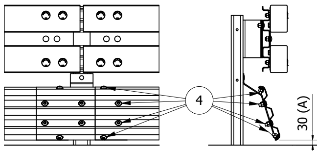
Fase "C" - Installazione nastri di protezione
