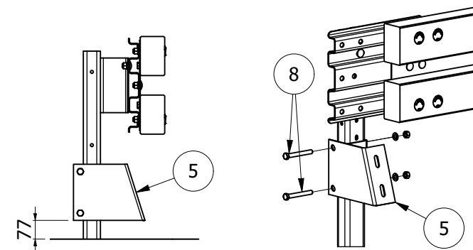
Installazione staffa terminale
