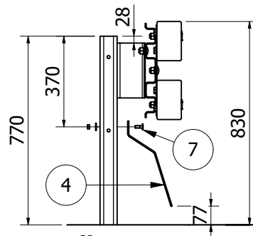
Fase "A" - Installazione staffa
