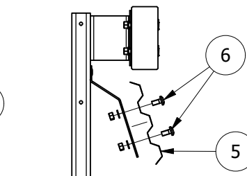
Fase "B" - Installazione piastra di continuità
