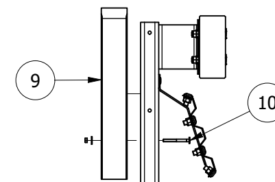
Riposizionamento guscio di protezione
