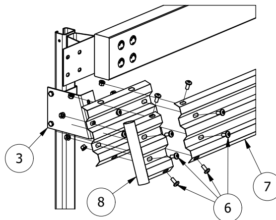
Fase "D" - Installazione terminale
