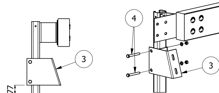
Installazione staffa terminale
