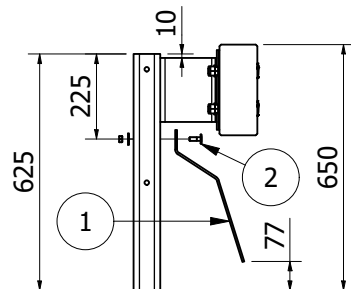
Fase "A" - Installazione staffa
