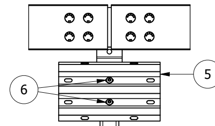
Fase "B" - Installazione piastra di continuità
