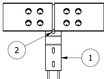
Fase "A" - Installazione staffa
