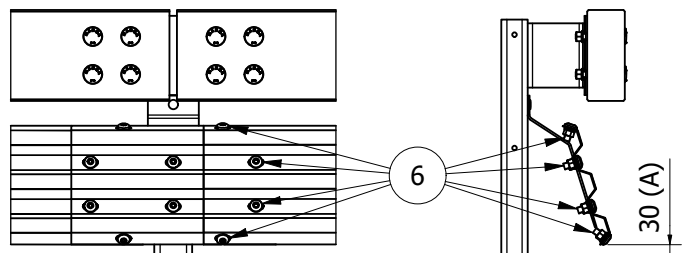
Fase "C" - Installazione nastri di protezione
