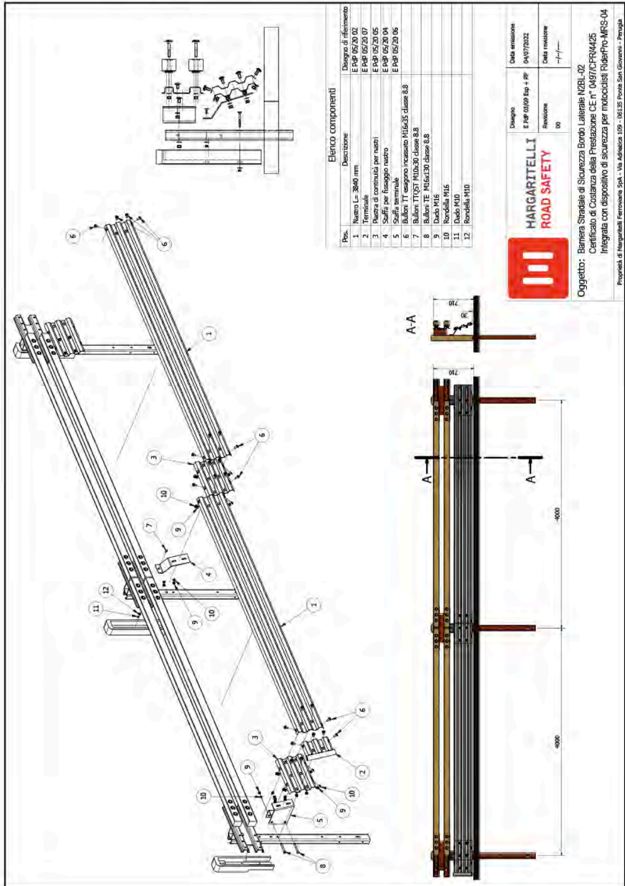
Figura 4 – Esploso del dispositivo, con indicazione dei singoli componenti
