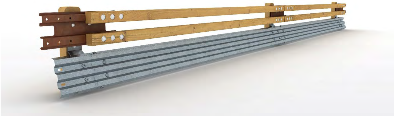
Figura 2 – dispositivo DSM RiderPro-MRS-04 integrato con N2BL-02
