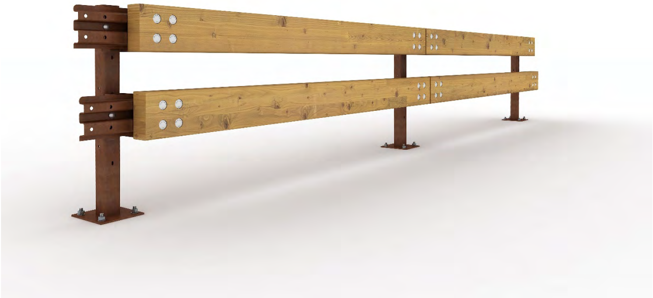
Figura 2 – Barriera senza rivestimento del montante
