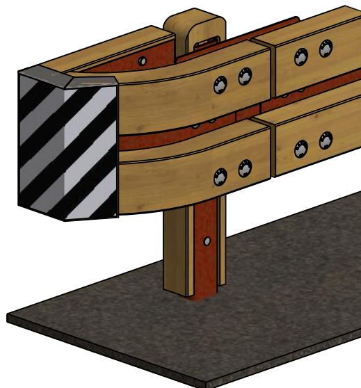
Soluzione con carter opzionale
