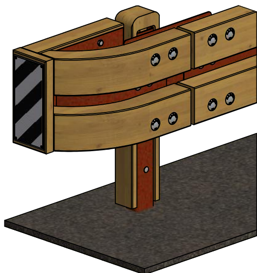
Soluzione con pannello frontale
