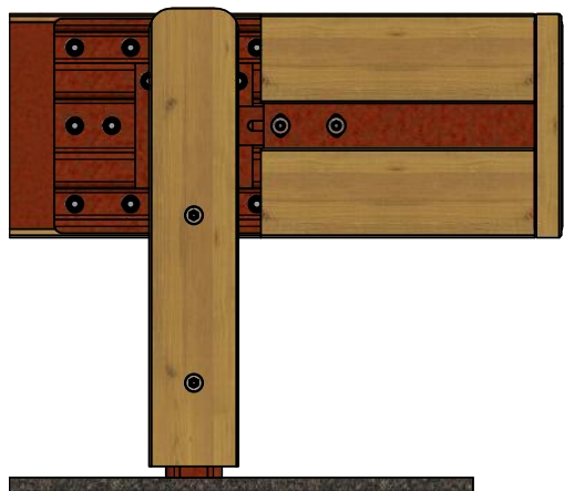
Vista posteriore
