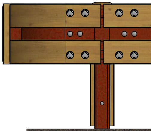
Vista longitudinale
